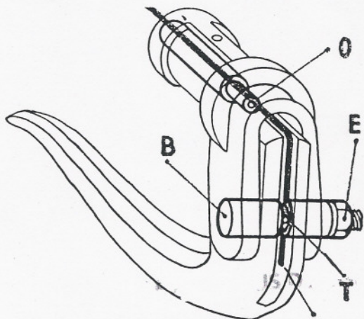
Fig. 14 Le Câble doit dépasser de 1 cm.
